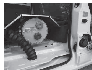
LPGタンクは 荷台に設置されます
